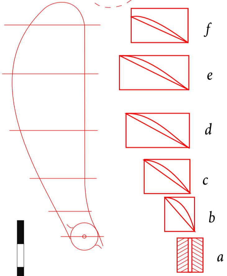
Fig. 6. Querschnitte. Nat. Grösse
